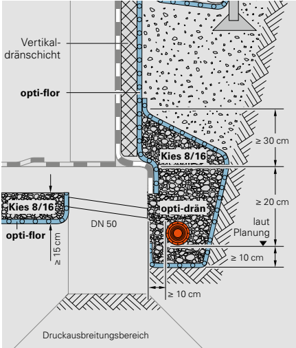
Querschnitt: Lage der Dränleitung
