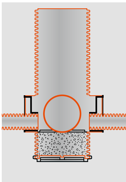
Sand-, Kies- oder Betonfüllung zur Erhöhung der Standsicherheit und als Auftriebssicherung
